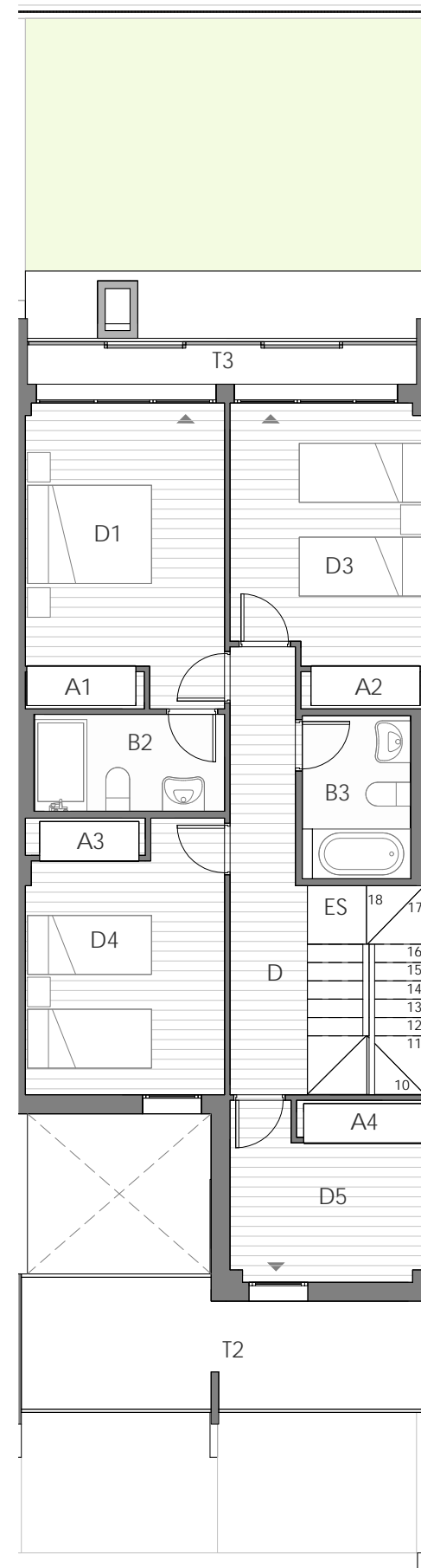
VIVIENDA C - PLANTA PRIMERA
