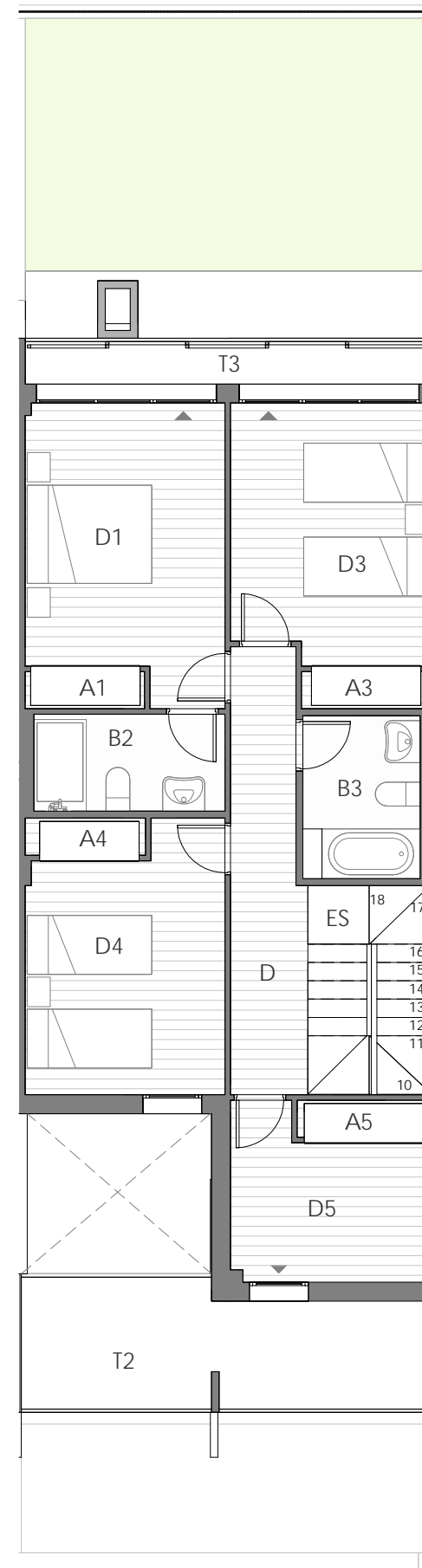
VIVIENDA B - PLANTA PRIMERA
