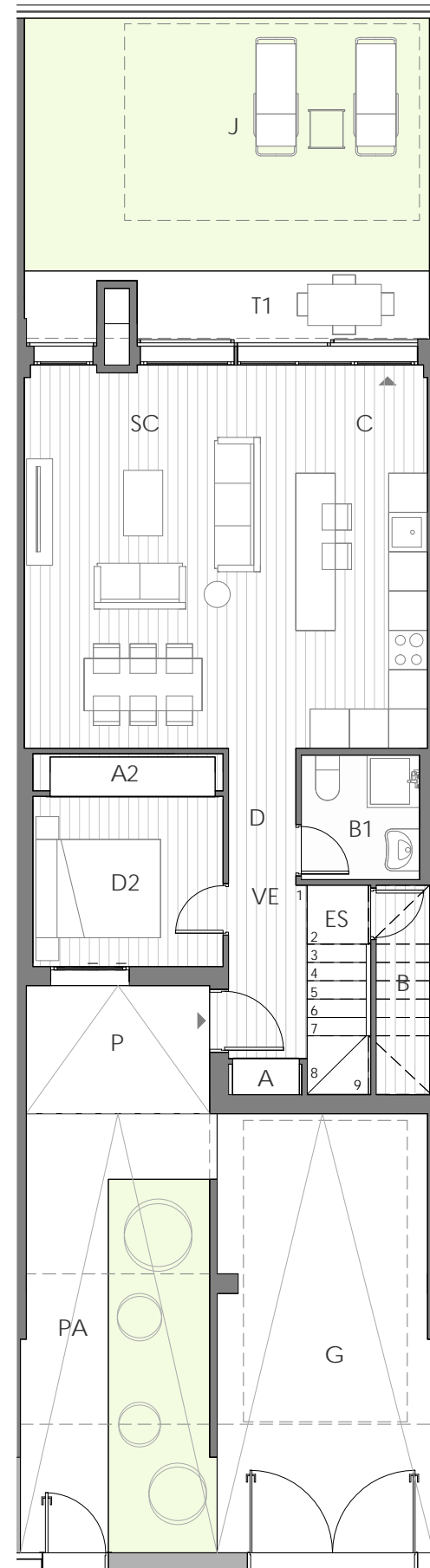
VIVIENDA B - PLANTA BAJA
