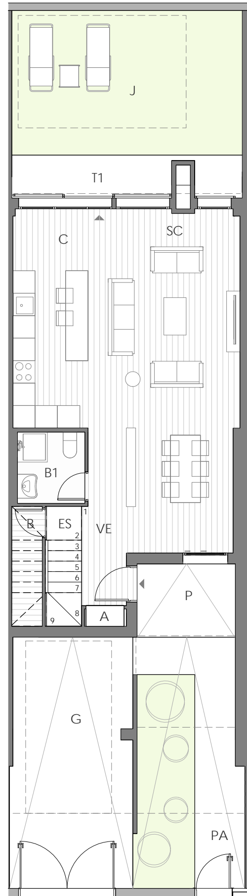
VIVIENDA D - PLANTA BAJA
