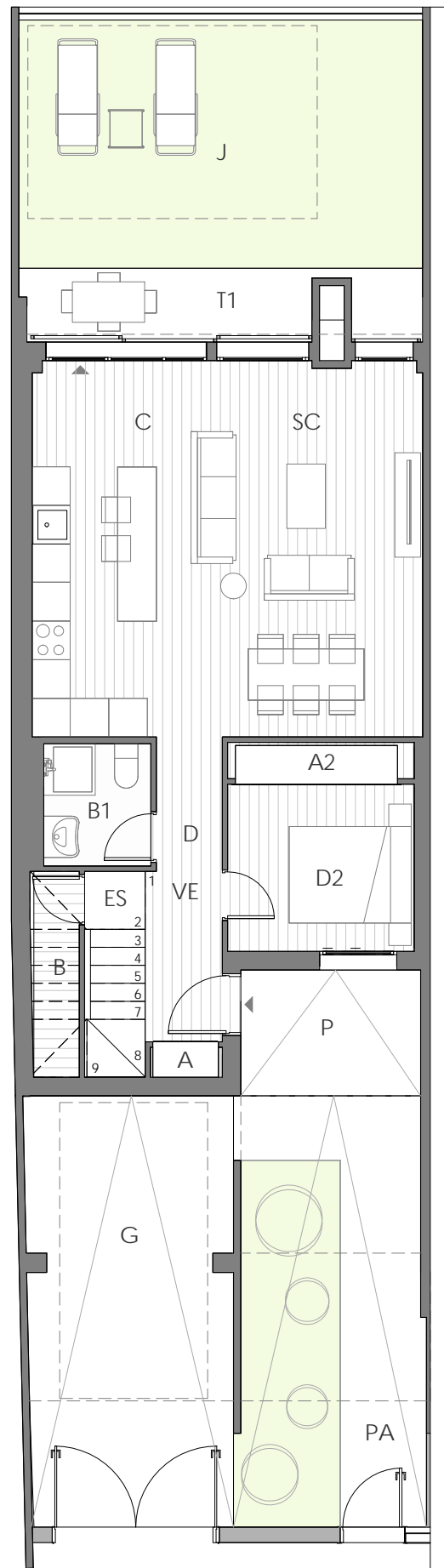
PLANTA BAJA
