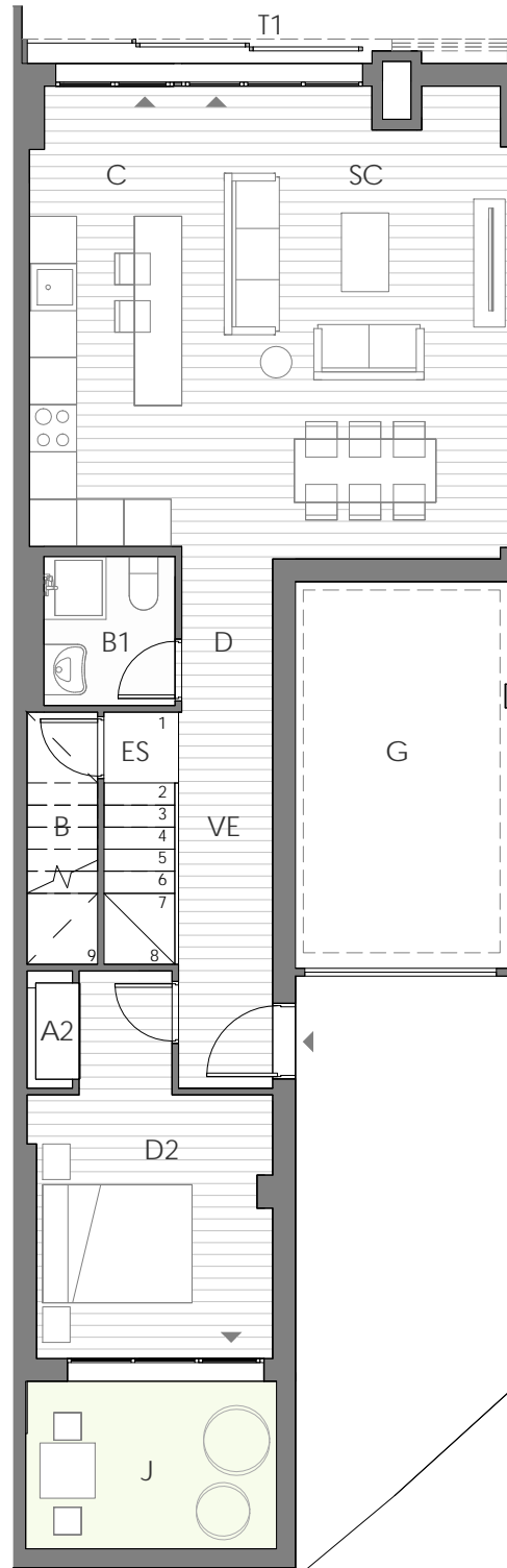
VIVIENDA E - PLANTA BAJA
