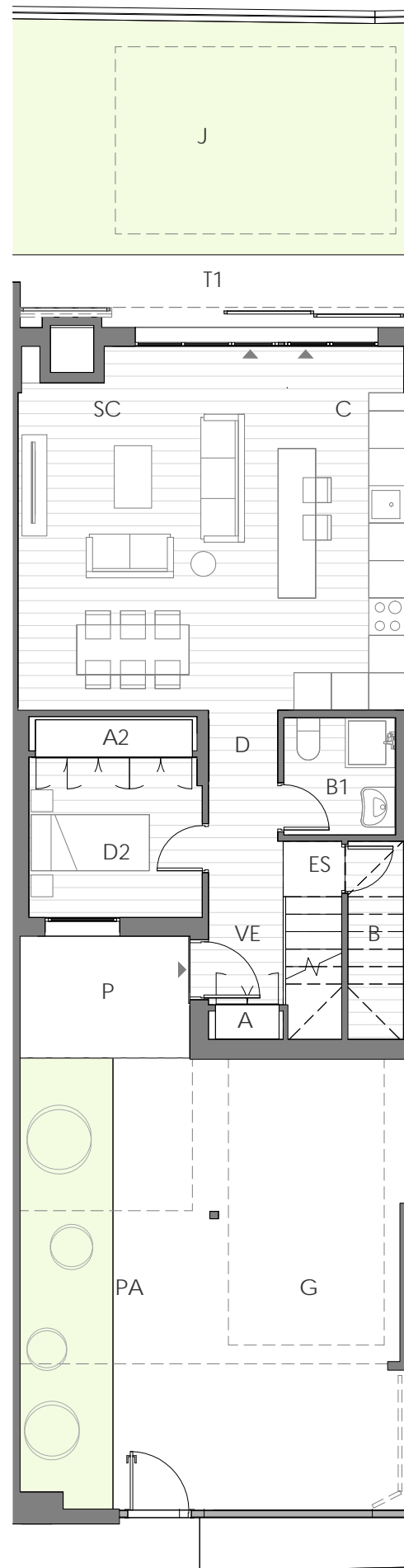
VIVIENDA B - PLANTA BAJA
