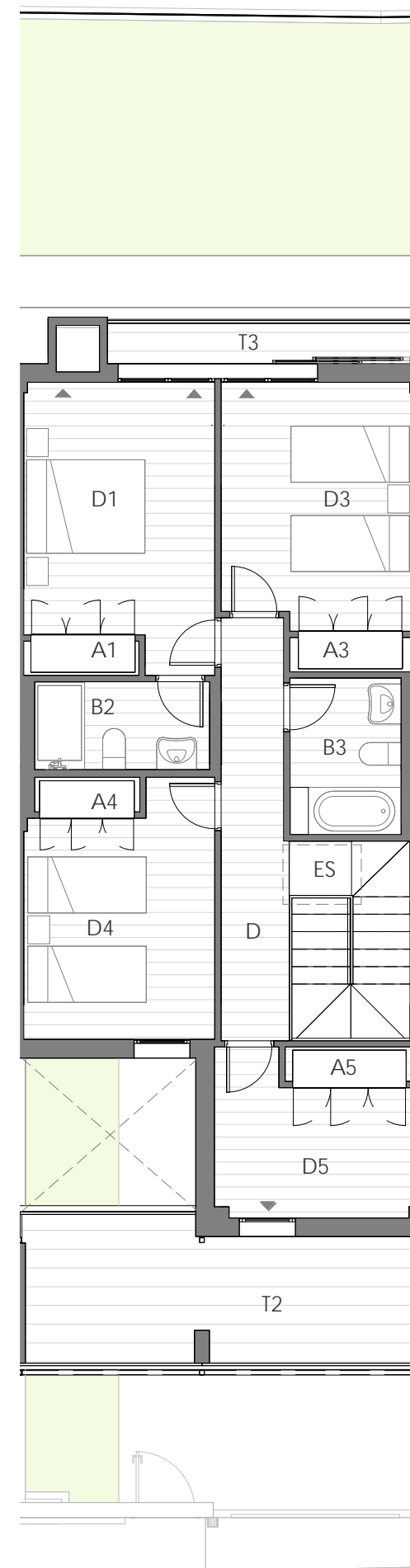
VIVIENDA B - PLANTA PRIMERA
